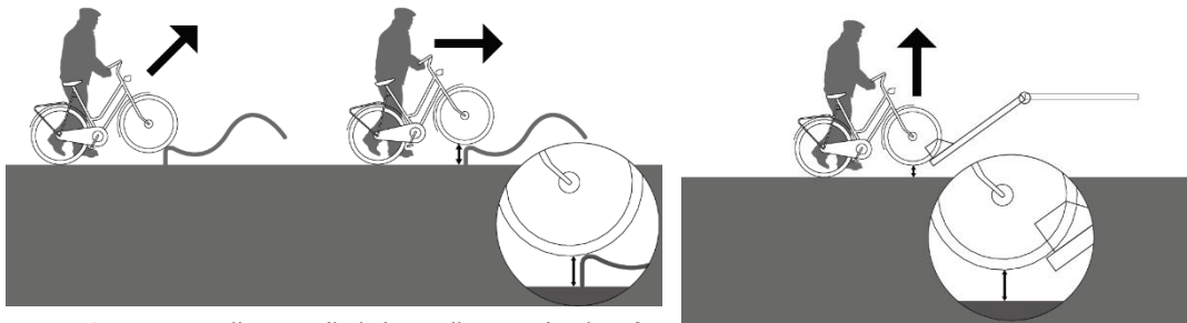
Figuur 3.1: Drempelhoogte (links) en tilhoogte (rechterfi-guur)
